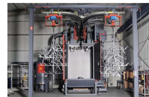
Κατεργασία με ατσαλοβολή
